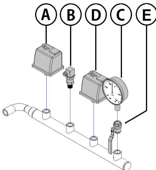
Рисунок 9 – Схема монтажа КИП
