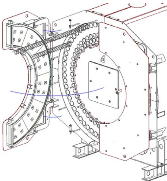
Рисунок 11 – Расположение турбулизаторов
