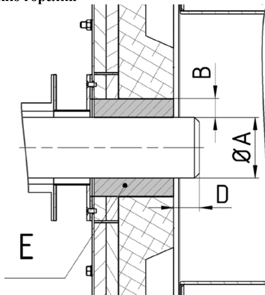
Рисунок 6 – Схема смонтированной во фронтную дверь горелки
