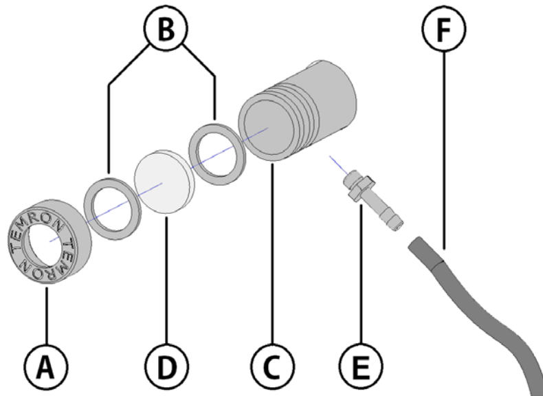
Рисунок 7 – Схема смотрового окошка (гляделки) котла
