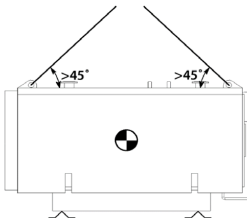
Рисунок 3 – Схема строповки и установки.
