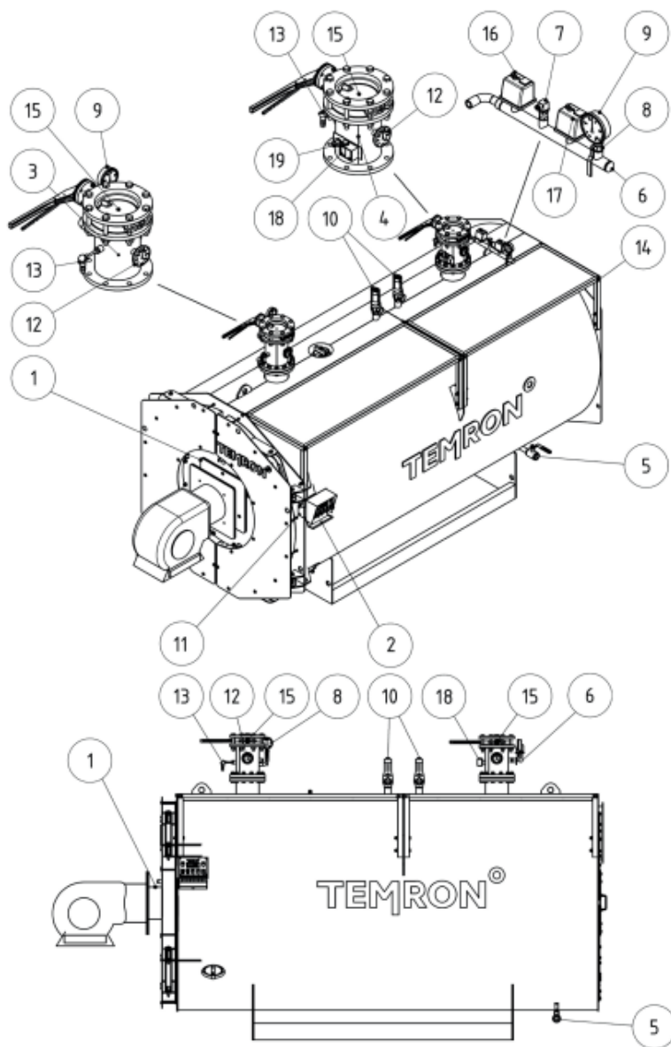
Рисунок 2 – Схема расположения дополнительного оборудования котла
