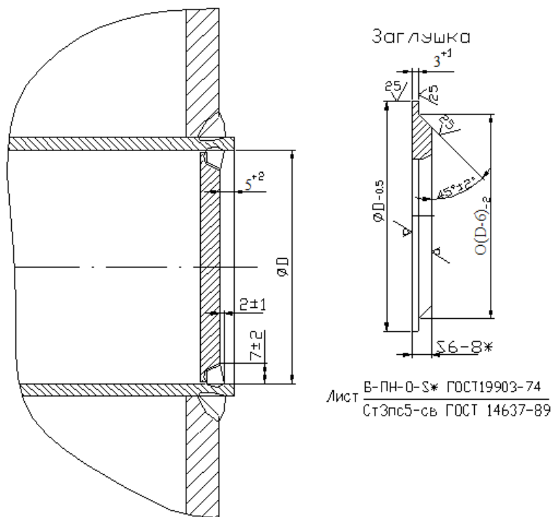
Рисунок 10 – Установка заглушки на дымогарную трубу
