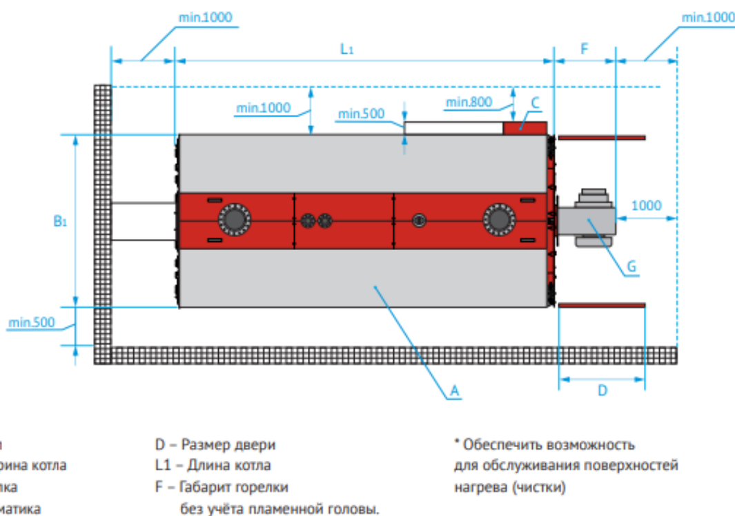
Рисунок 4 – Схема рекомендуемого расположения котла в помещении
