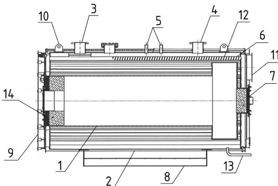
Рисунок 1 - Продольный разрез водогрейного котла серии WH
