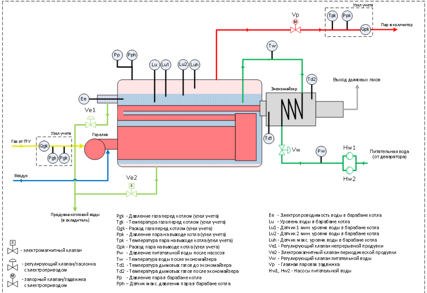
Типовая схема автоматизации парового котла с автоматизированной горелкой
